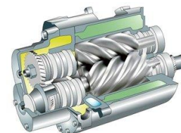
šroubový element
